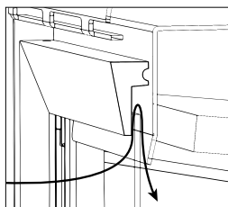
Entrée d'air secondaire sans régulation
