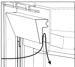
Entrada de ar secundário sem regulação
